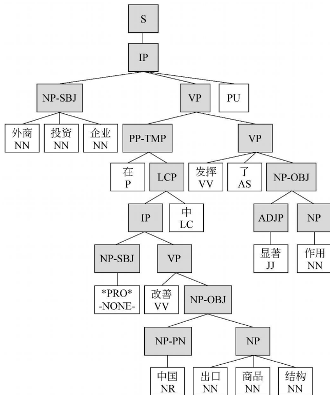
图 1 PennCT 短语结构树示例
